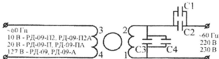
Рисунок 3 – Схема электрическая включения двигателей на напряжение 220 или 230 В частотой 60 Гц в комплекте с конденсаторами С1 и С3 типа МБГТ-1000 В-0,1 мкФ±10%, С2 и С4 типа МБГЧ-1-2А-500-0,25±10%.
