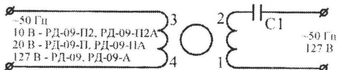
Рисунок 1 – Схема электрическая включения двигателей на напряжение 127 В частотой 50 Гц в комплекте с конденсатором С1 типа МБГТ-300 В-1 мкФ \pm 10%.
