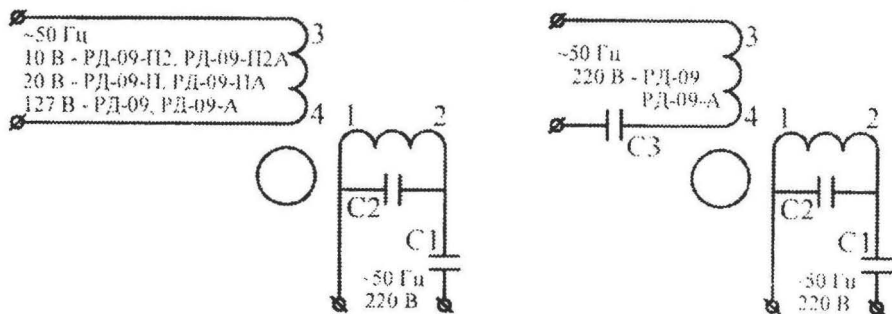
Рисунок 2 – Схема электрическая включения двигателей на напряжение 220 В частотой 50 Гц в комплекте с конденсаторами С1 и С3 типа МБГЧ-1-2А-500-0,5 \pm 10%, С2 типа МБГЧ-1-2А-250-0,5 \pm 10%.
